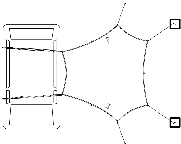
▲車とタープ本体を上から見た図
