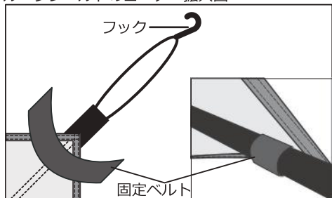
ルーフシールドのコーナー拡大図
